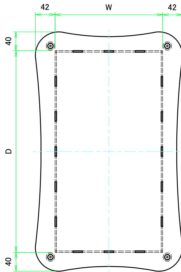
上カバー / Top cover
