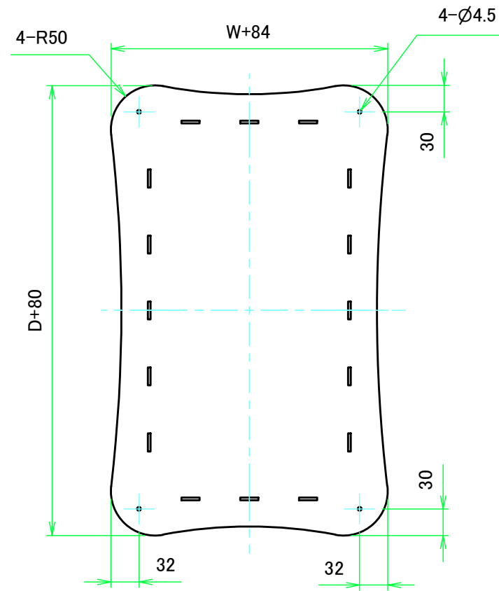
上カバー表面 / Top cover Frontside
